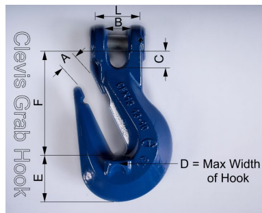
Clevis grab hook
